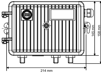
Dimensions VX 26 H 0650
