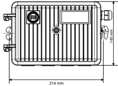
Dimensions VX 29 H 0650
